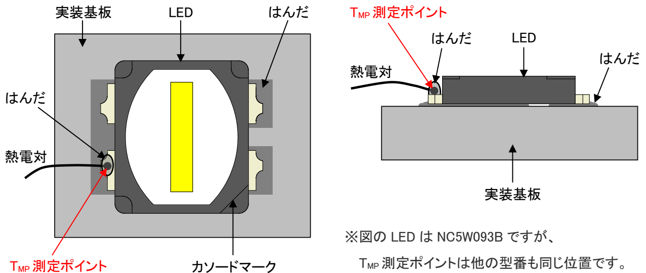
図 1. T_{MP} 測定ポイント
