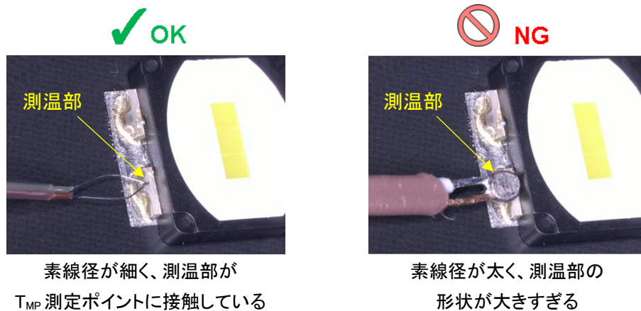
図 2. 熱電対取り付けの例(はんだ付け前)
